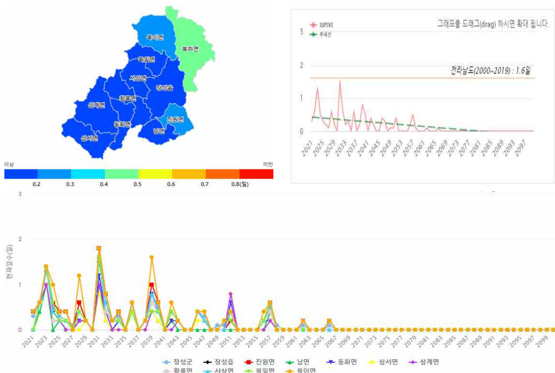
[표Ⅲ.1 -14] 한파일수, SSP5-8.5, 장성군, 2021~2100년(연별)
