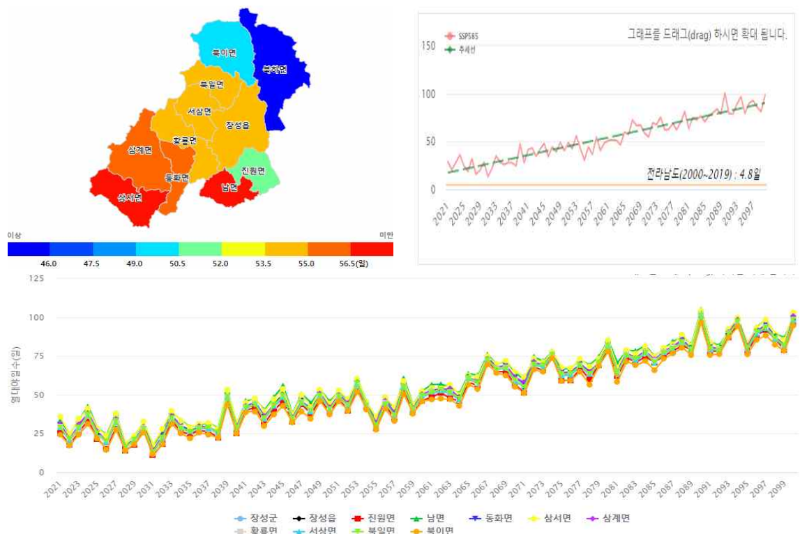
[표Ⅲ.1 -13] 열대야일수, SSP5-8.5, 장성군, 2021~2100년(연별)
