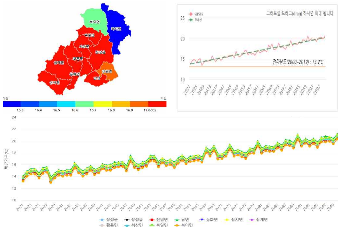
[표Ⅲ.1 - 8] 평균기온, SSP5-8.5, 장성군, 2021~2100년(연별)
